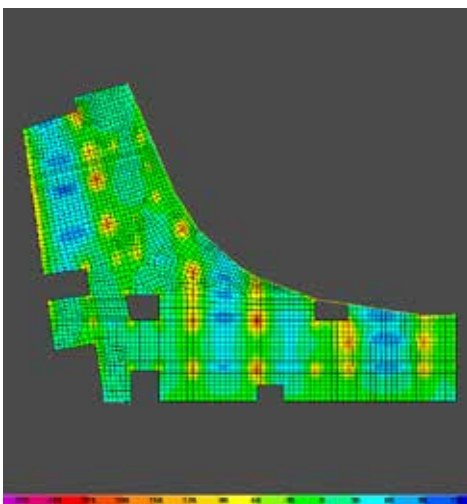
Modelo de cálculo (SAP 2000) — Aerogare
